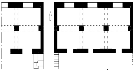
الصور (15)، (16): توضح طريقة تصميم بناء المسكن التقليدي في الباعج.
